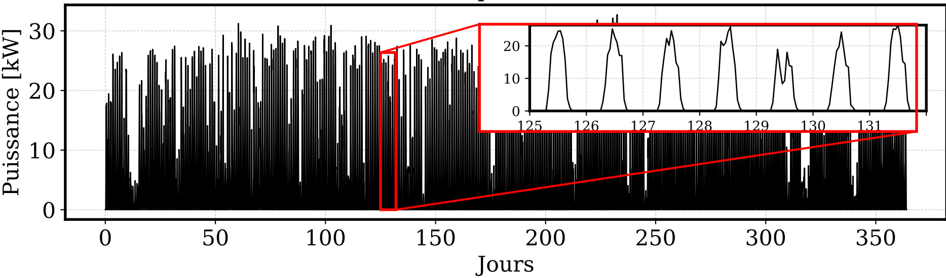
Profil de production PV
